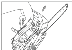
Остановка цепи тормозом цепи
