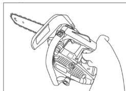
Запуск двигателя ручкой стартера
